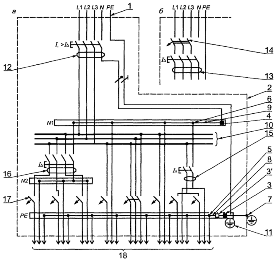
1 — питающая цепь; 2 — проводящая оболочка щитка; 3, 4 — зажимы проводников ввода (нулевого защитного PE и нулевого рабочего N); 3' — неиспользованный зажим (назначение согласно рисунку А.3); 5, 6 — зажимы для нулевого защитного PE и нулевого рабочего N проводников групповой цепи; 7 — зажим для присоединения заземляющего проводника (см. рисунок А.5) или проводника уравнивания потенциалов; 8 — соединительный элемент зажимов нулевых защитных проводников PE (ввода, поз. 3 и групповых цепей, поз. 5); 9 — соединительный элемент зажимов нулевых рабочих проводников N (ввода, поз. 4 и групповых цепей, поз. 6); 10 — соединительные элементы входных выводов защитных аппаратов групповых цепей или сборные шины; 11 — знак заземления у зажимов (поз. 3, 7); 12 — устройство защитного отключения на вводе щитка по варианту а); 13, 14 — устройство защитного отключения и выключатель на вводе щитка по варианту б); 15, 16 — устройства защитного отключения групповых цепей; 17 — автоматический выключатель; 18 — линии групповых цепей
